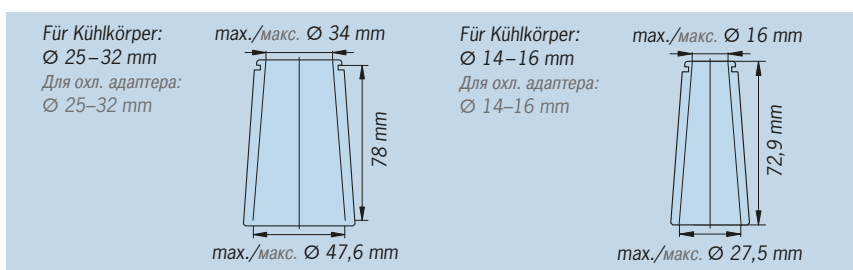
Kühlkörper mit Adapter für spezielle Schrumpffutter Охлаждающий адаптер с переходником для специальных термопатронов
